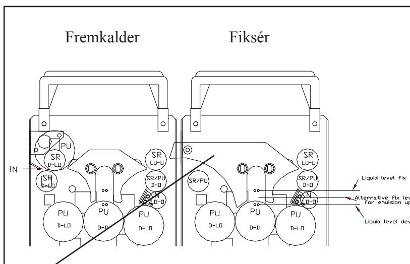
Racktegning R2 - placering af ny guide
