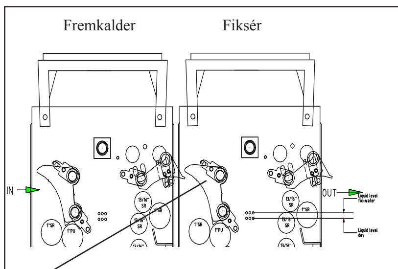
Racktegning R43 - placering af ny guide
